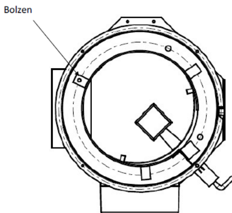
Abgas vorne
