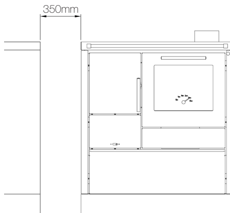
Montagebeispiel TR_B (ohne Brandschutzeinheiten)
