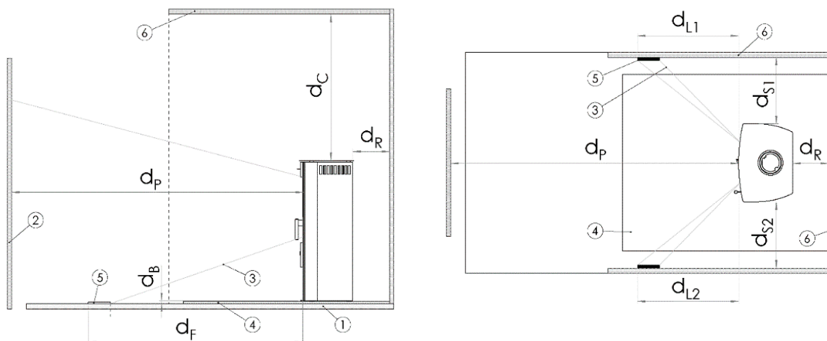
Abbildung 17 - Schematische Darstellung der Mindestabstände (siehe Tabelle 3)
