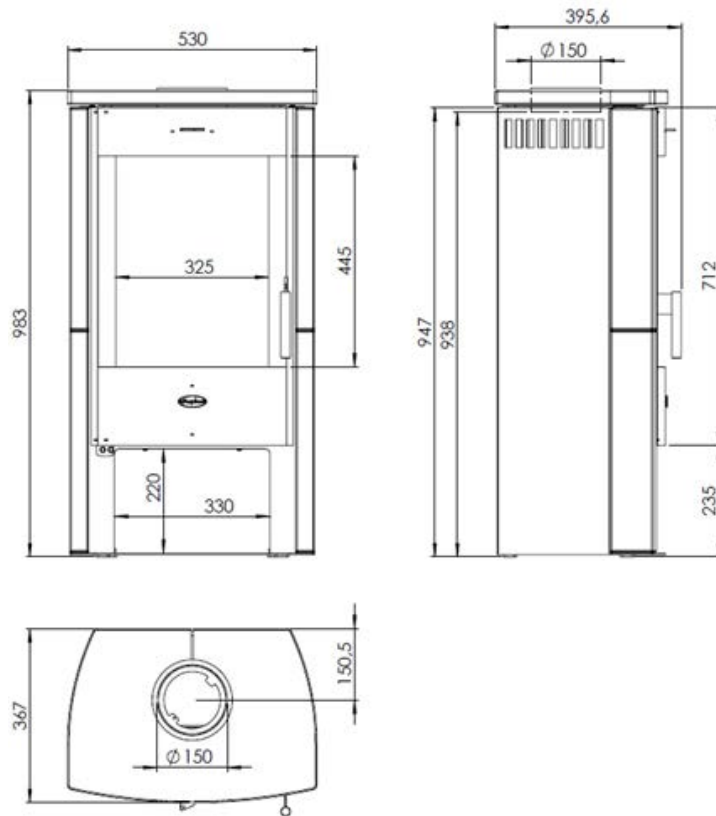
Abbildung 6 - Hauptmaße
