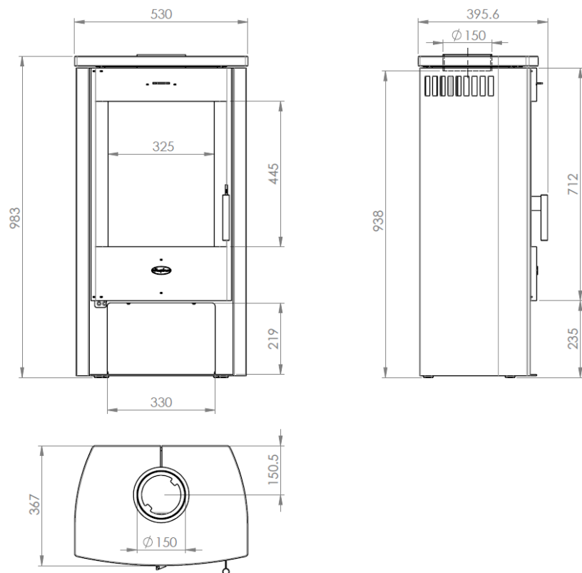
Abbildung 5 – Hauptmaße
