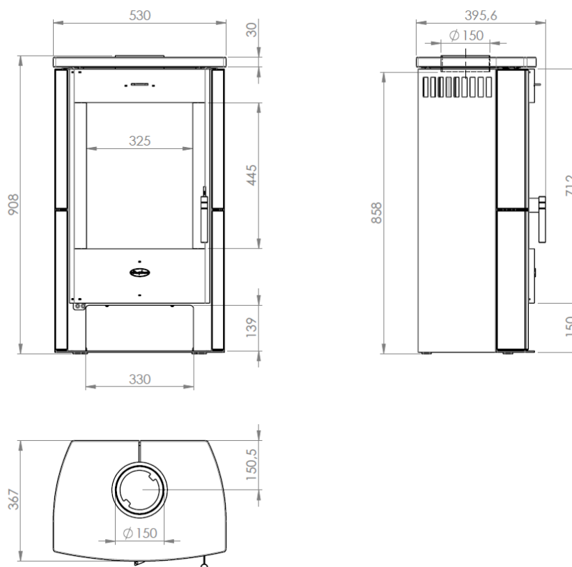
Abbildung 3 - Hauptmaße
