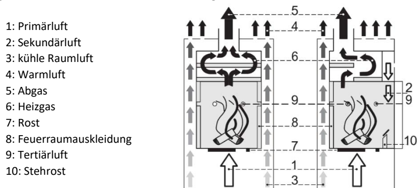
Abbildung 14 – Fire-Plus System, schematische Darstellung
