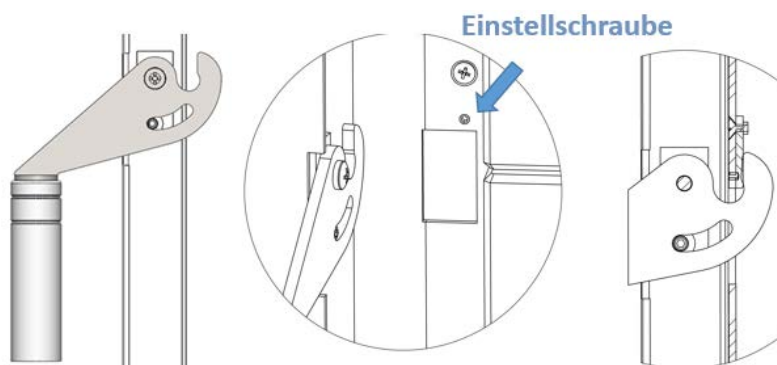
Abbildung 24 - Verriegelung der Tür
