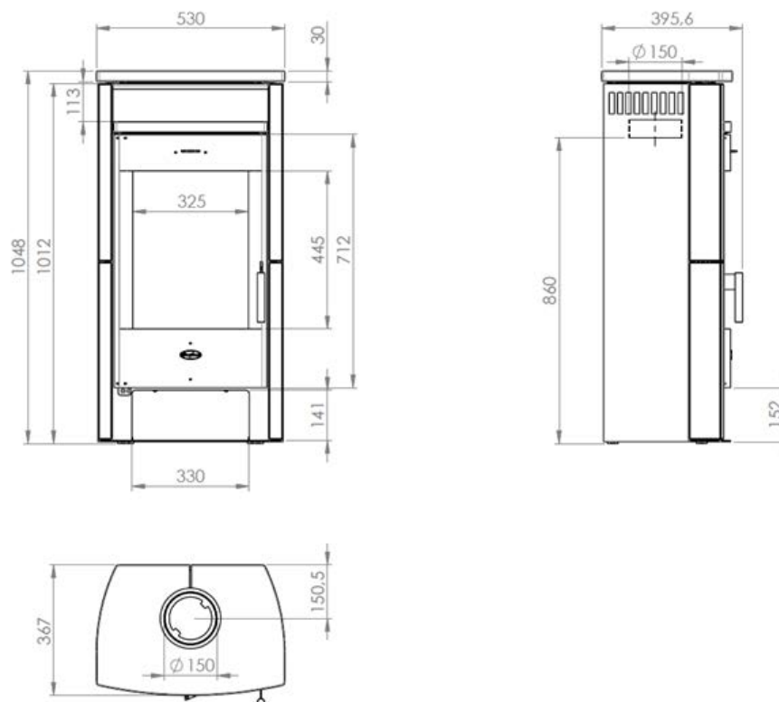
Abbildung 7 – Hauptmaße
