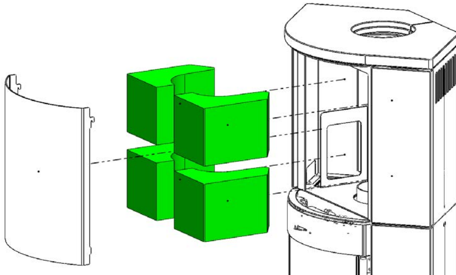
Abbildung 15 – Wärmespeichersteine M1590
