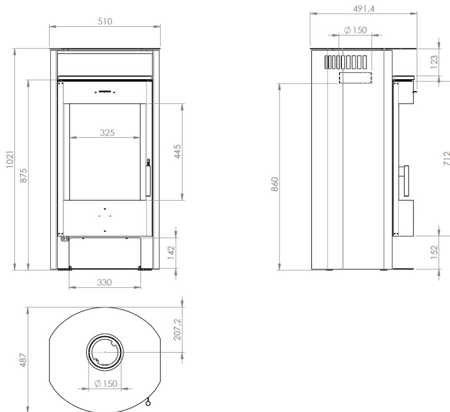
Abbildung 11 - Hauptmaße
