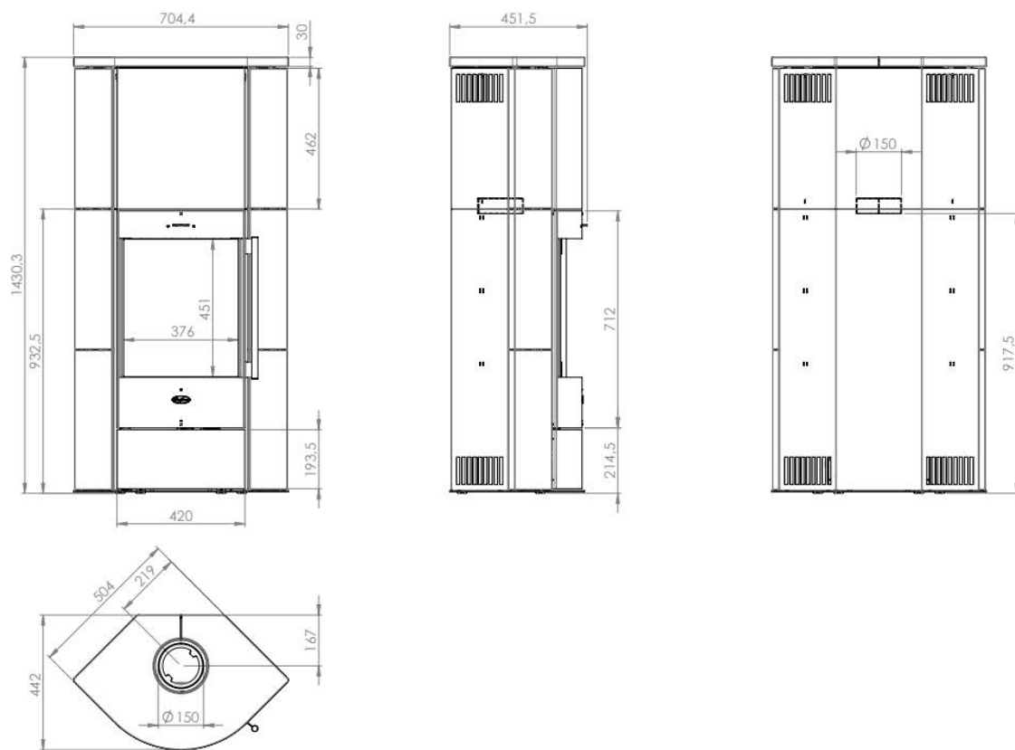
Abbildung 13 - Hauptmaße
