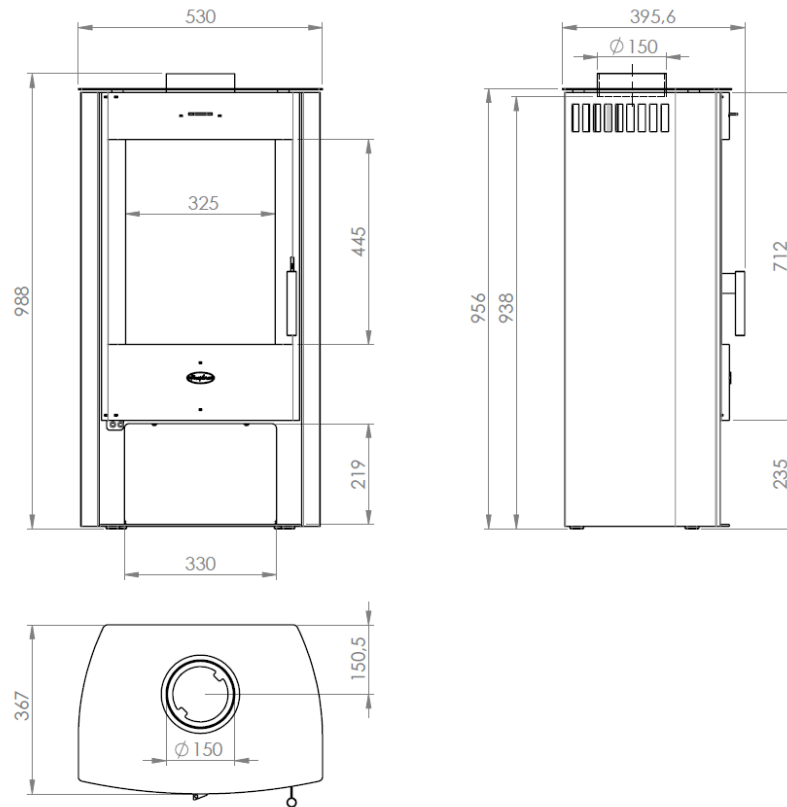
Abbildung 4 - Hauptmaße
