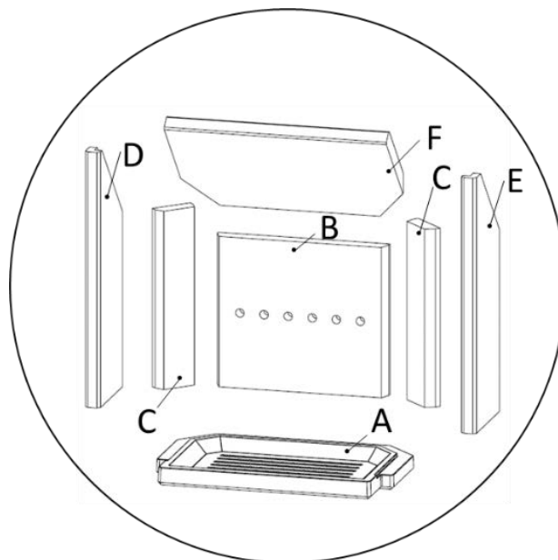
Abbildung 21 – Feuerraumaukleidung mit Rost
