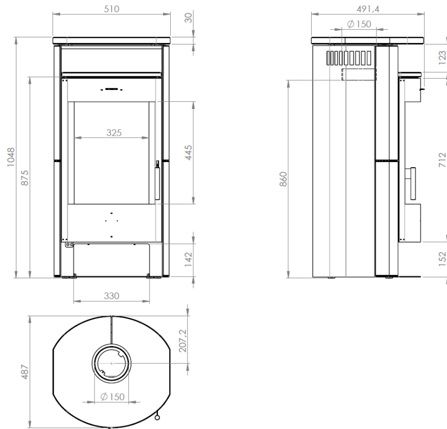
Abbildung 10 - Hauptmaße
