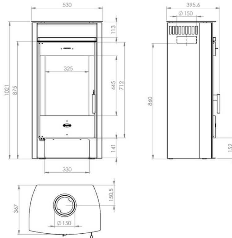
Abbildung 8 - Hauptmaße
