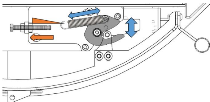
Abbildung 23 – Schnappverschluss
