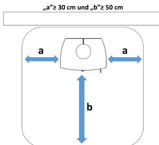
Abbildung 16- Bodenplatte
