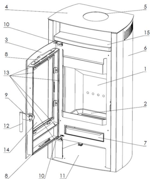
Abbildung 1 – Aufbau des Geräts
