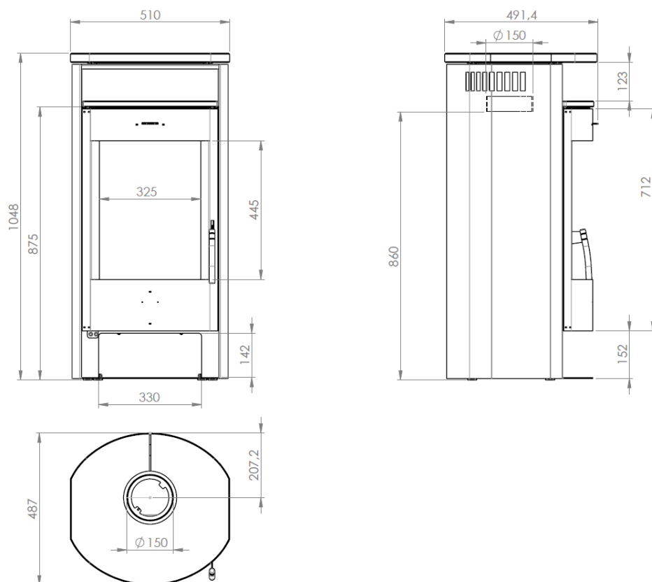
Abbildung 12 - Hauptmaße
