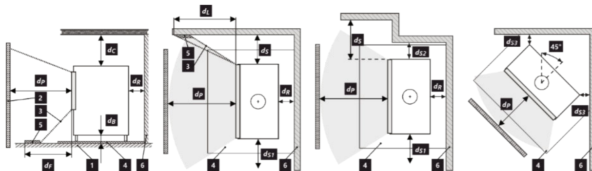
Abb. 2 Abstand zu brennbaren Materialien
