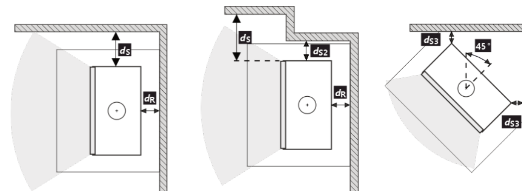
Fig. 3 Distance de sécurité du produit aux matériaux non-combustibles
