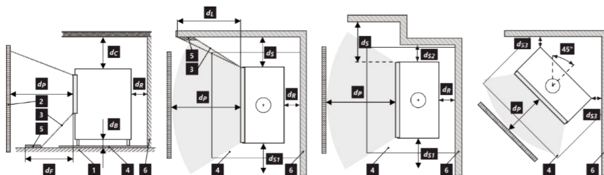
Fig. 2 Distance de sécurité du produit aux matériaux
