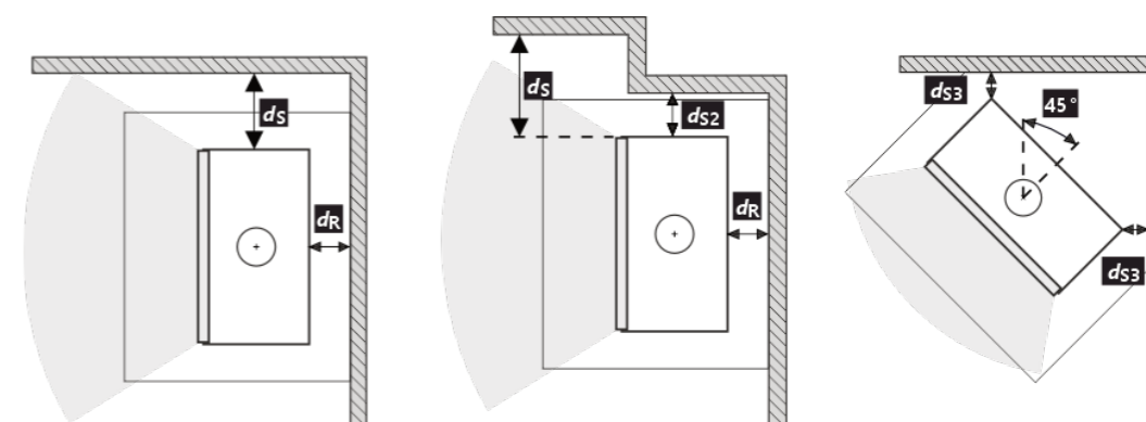
Fig. 3 Distanza di sicurezza da materiali non infiammabili sono
