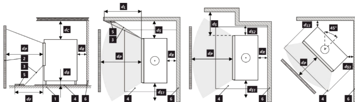
Fig. 2 Distanza di materiali infiammabili
