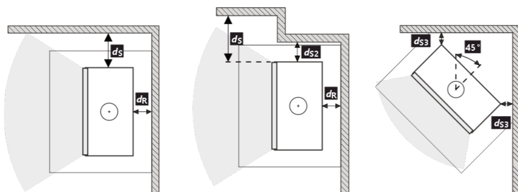
Abb. 3 Abstand zu nicht brennbaren Materialien
