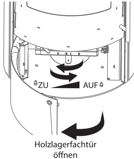
Abb.2.3 Verbrennungsluftschieber (schematische Darstellung)
