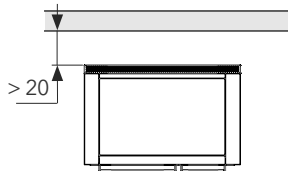
ohne Brandschutzeinheiten
