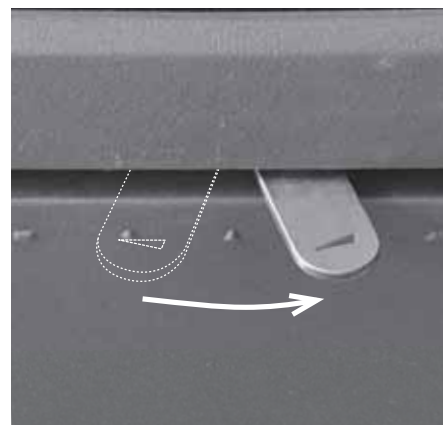
Abb. 4.19 Luftschieber ganz rechts, Anheizstellung und Betriebsstellung bei Speicherleistung
