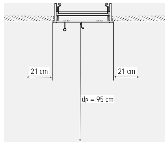
Abb. 2.2 DIAMANT H13.2: Strahlungsbereich der Gerätefront – schematische Darstellung
