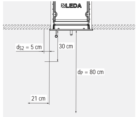
Abb. 2.1 DIAMANT H10.2 und DIAMANT H20.2: Strahlungsbereich der Gerätefront – schematische Darstellung
