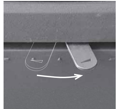
Abb. 4.11 Luftschieber ganz rechts, Anheizstellung
