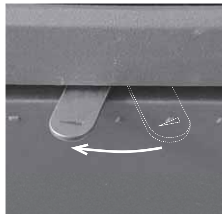
Abb. 4.17 Luftschieber ganz links, Verbrennungsluft geschlossen
