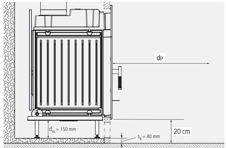
Abb. 2.3 Strahlungsbereich der Front – schematische Darstellung Seitenansicht
