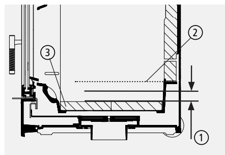
Abb. 4.23 Aschebett, Ascheniveau
