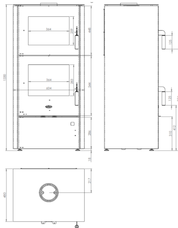
Abbildung 2 – Hauptmaße
