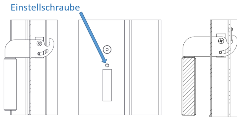
Abbildung 14 – Verriegelung der Tür
