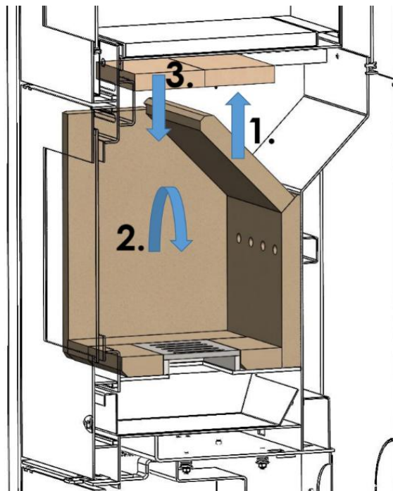
Abbildung 13 – Zugang zum Rauchraum
