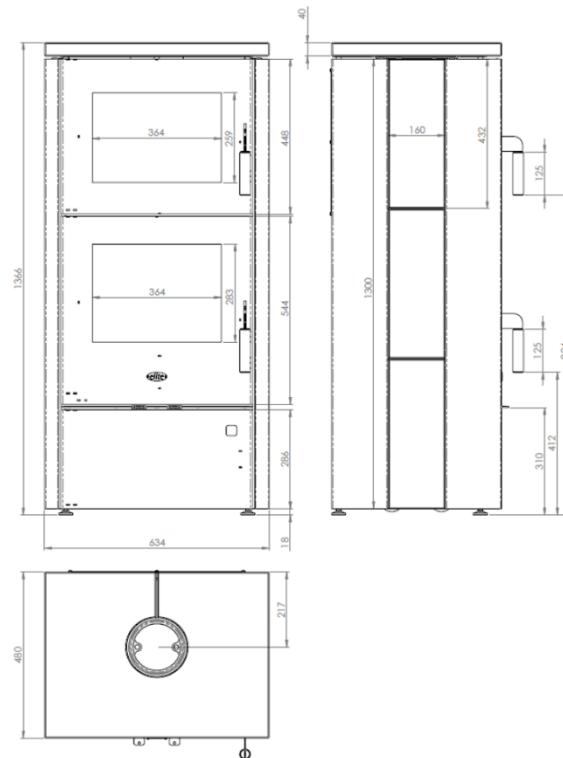
Abbildung 3 - Hauptmaße
