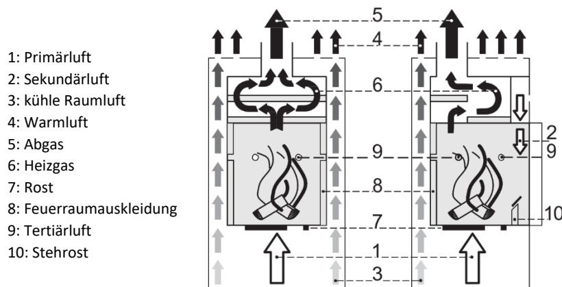
Abbildung 4 – Fire-Plus System, schematische Darstellung
