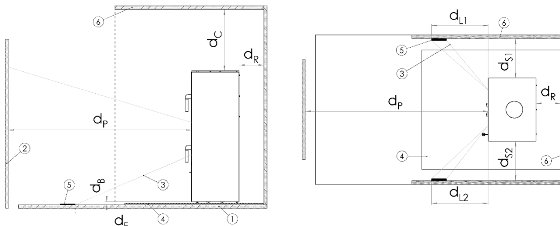
Abbildung 7 - Schematische Darstellung der Mindestabstände (siehe Tabelle 2)
