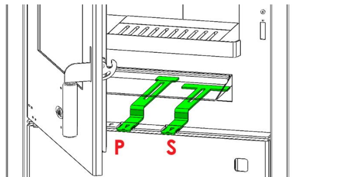
Abbildung 10 - P: Primärluftregler, S: Sekundärluftregler
