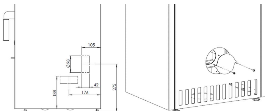
Abbildung 5- Verbrennungsluftanschluss
