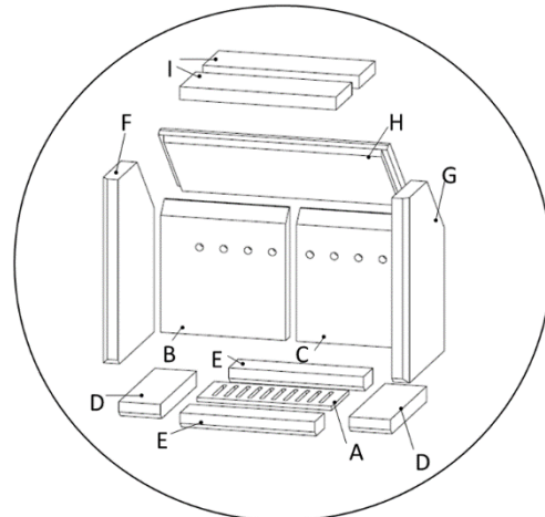
Abbildung 12 – Feuerraumauskleidung mit Rost
