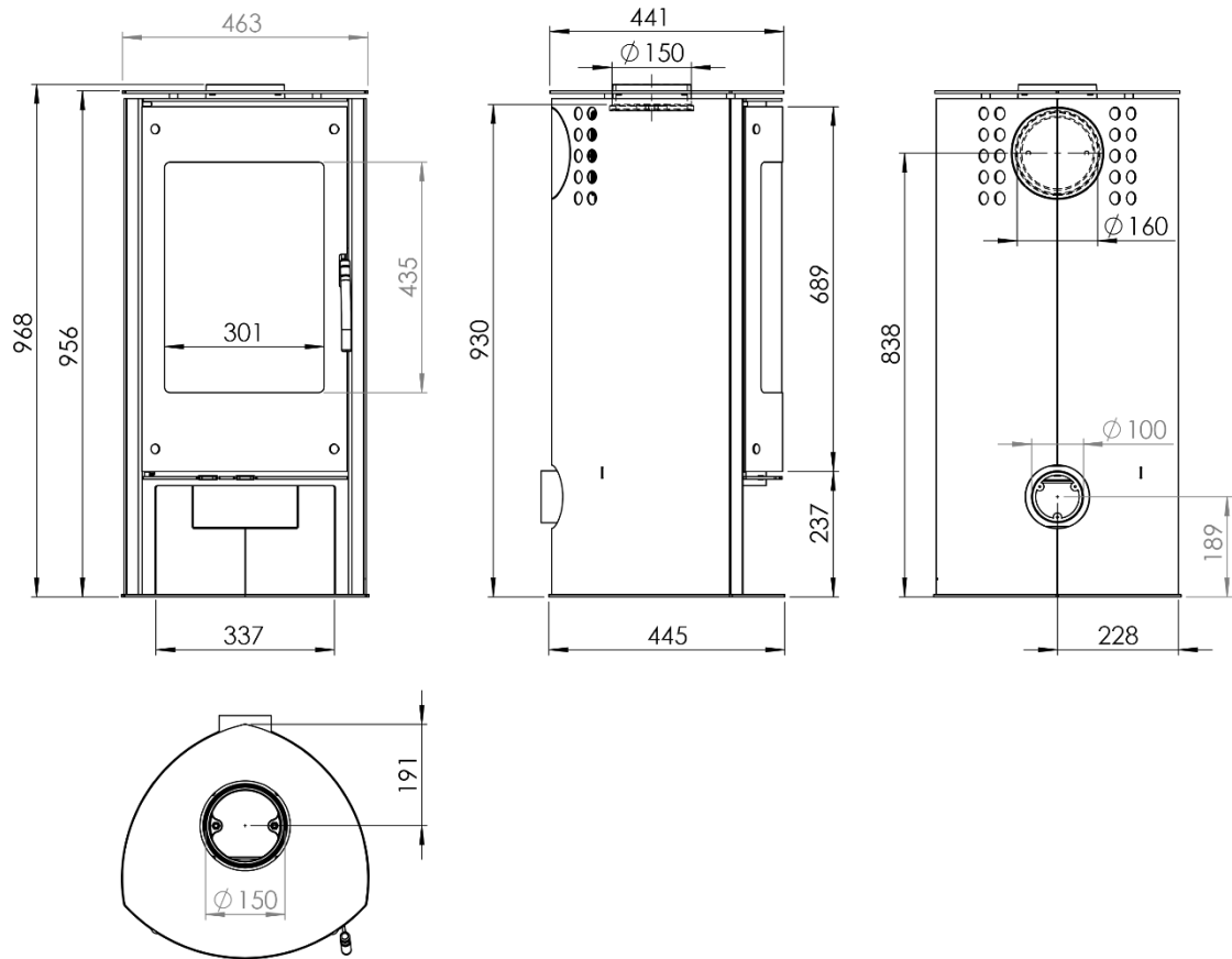
Abbildung 4 – Hauptmaße
