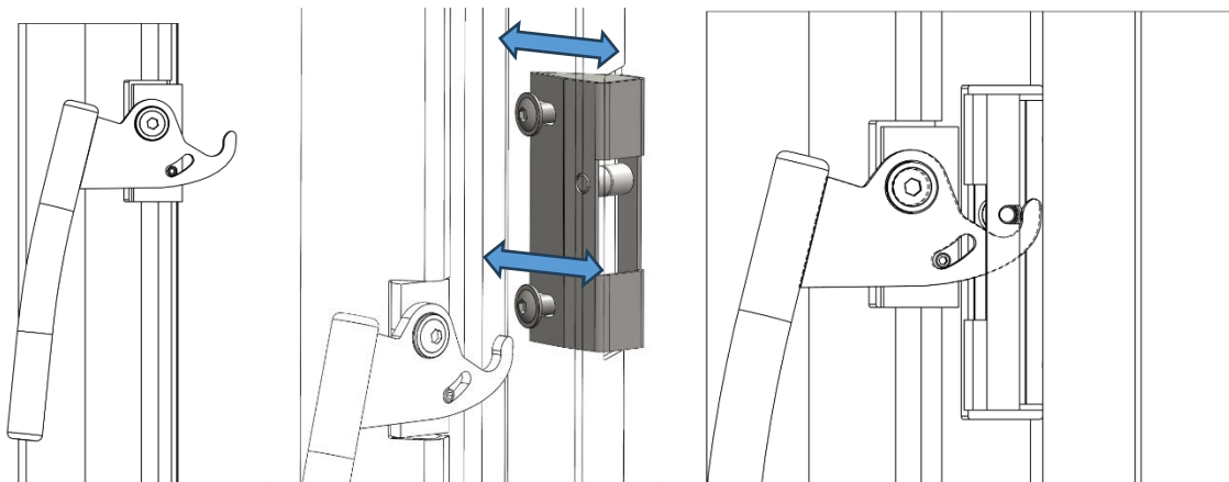
Abbildung 16 - Türverschluss
