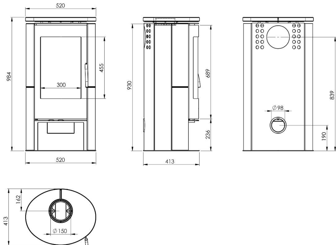
Abbildung 3 - Hauptmaße
