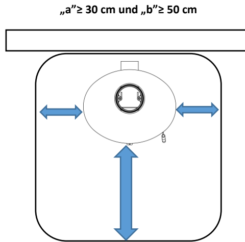
Abbildung 9 - Bodenplatte
