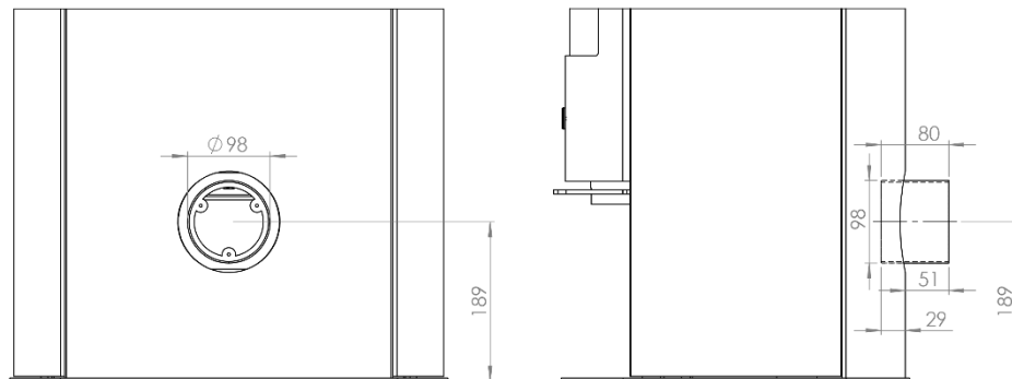
Abbildung 8- Verbrennungsluftanschluss
