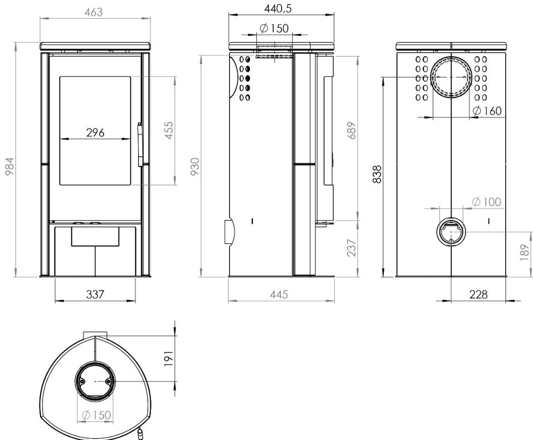
Abbildung 5 - Hauptmaße
