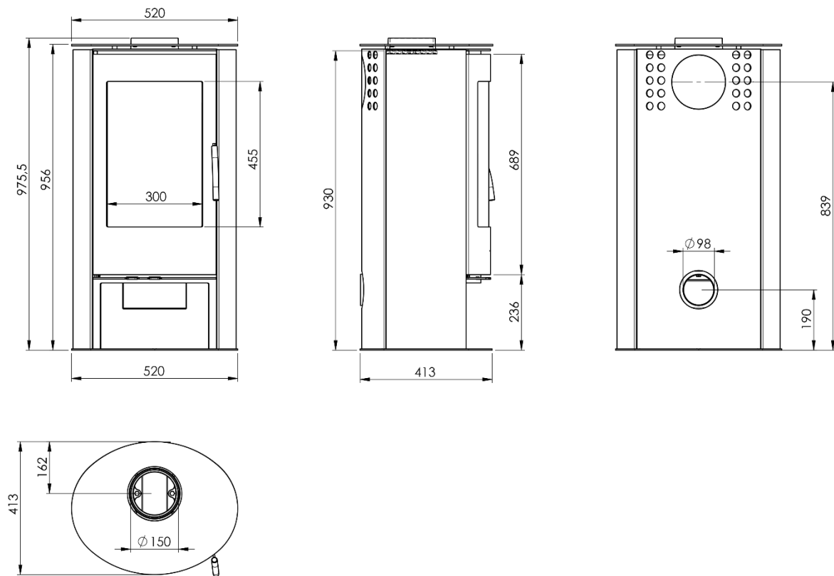
Abbildung 2 - Hauptmaße
