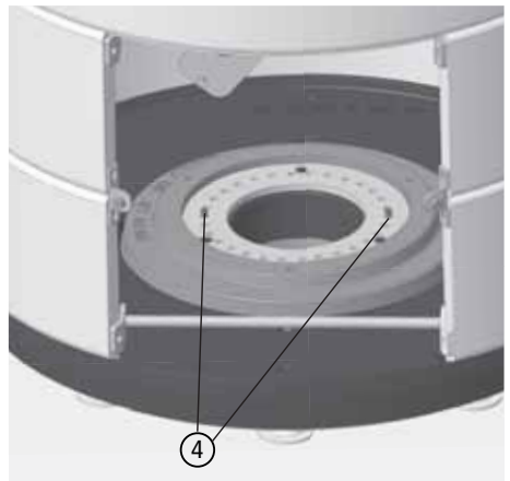
Abb. 3.13 Anschlag-Stifte, Einstellen des linken und rechten Endanschlags
