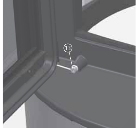
Abb. 3.29 gespannte Türfeder
