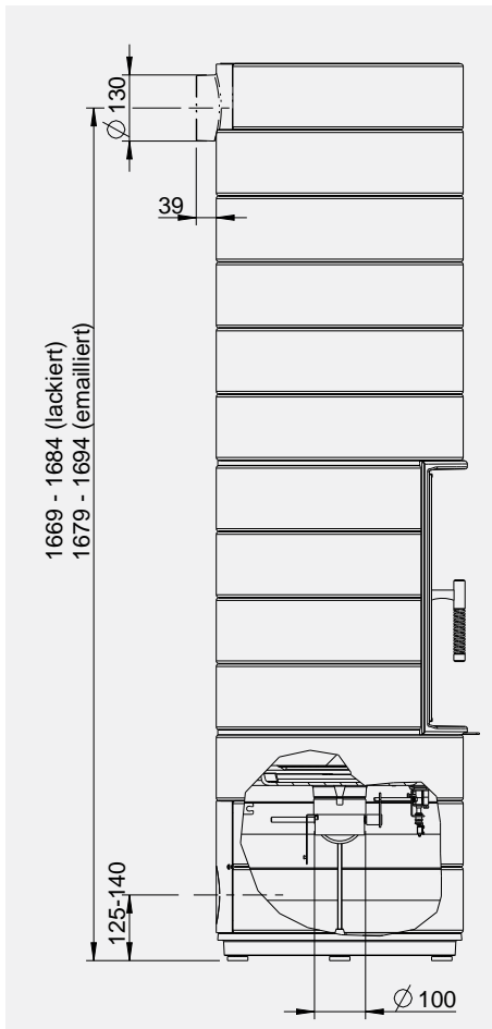
Abb. 3.47 Abgasanschluss bei COLONA lite mit 6 Gussringen
