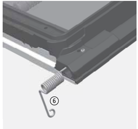
Abb. 3.25 Türfeder einsetzen
