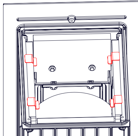
Abb. 10: Halter aufgelegt
