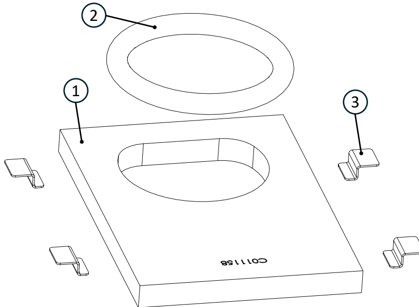
Abb. 6: Überblick Brennraumdeckel
