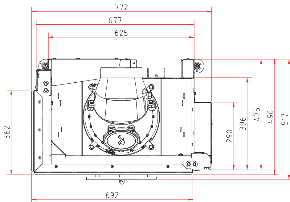
Draufsicht M 1:10
