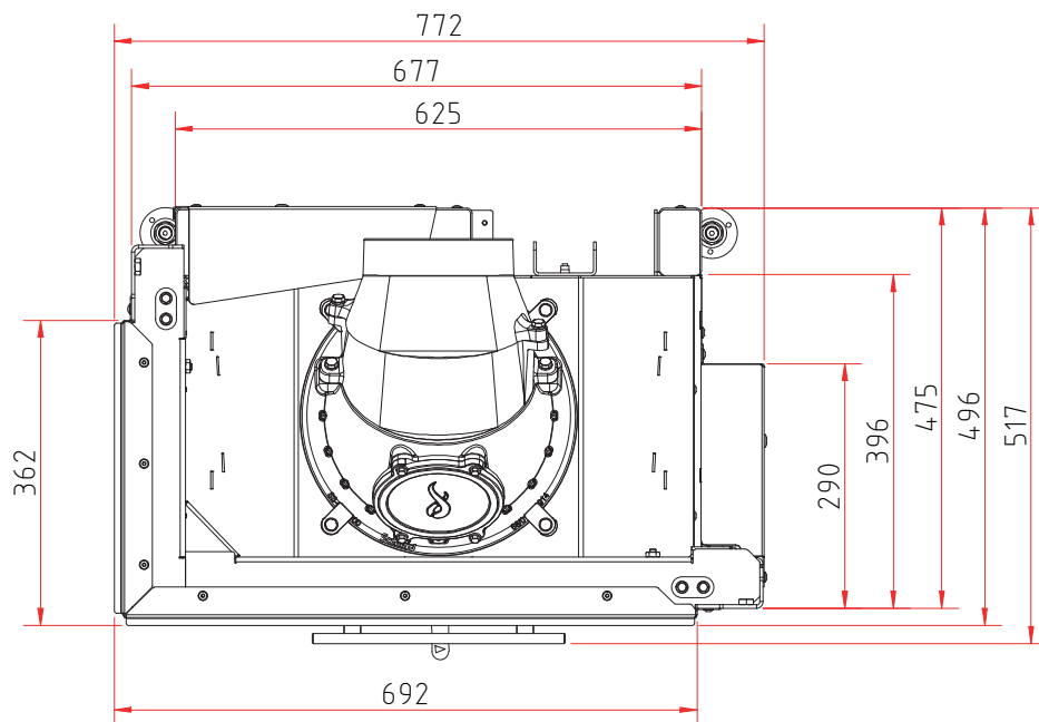
Draufsicht M 1:10
