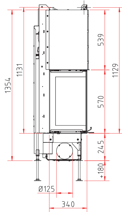
Seitenansicht M 1:20
