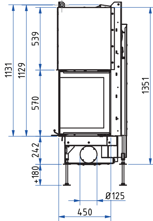
Seitenansicht M 1:20
