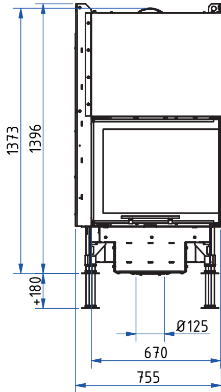
Frontansicht M 1:20
