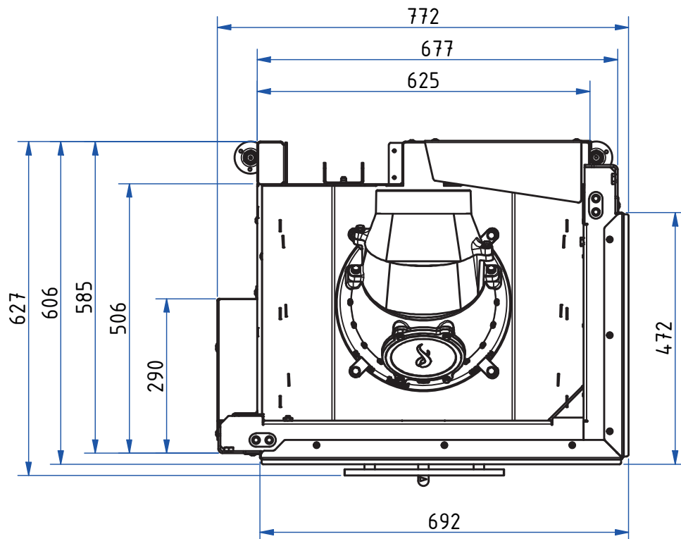
Draufsicht M 1:10
